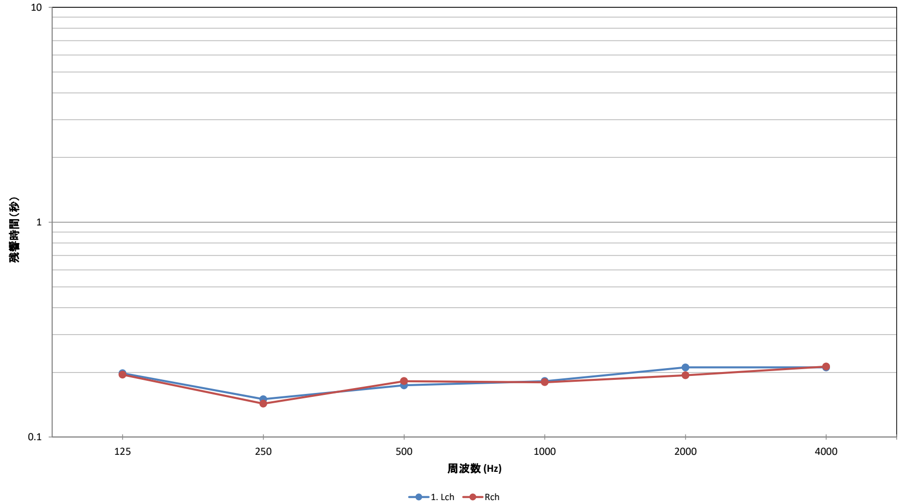
東京都文京区N.N様邸 残響時間周波数特性 (測定位置リスニングポイントH=1000)
