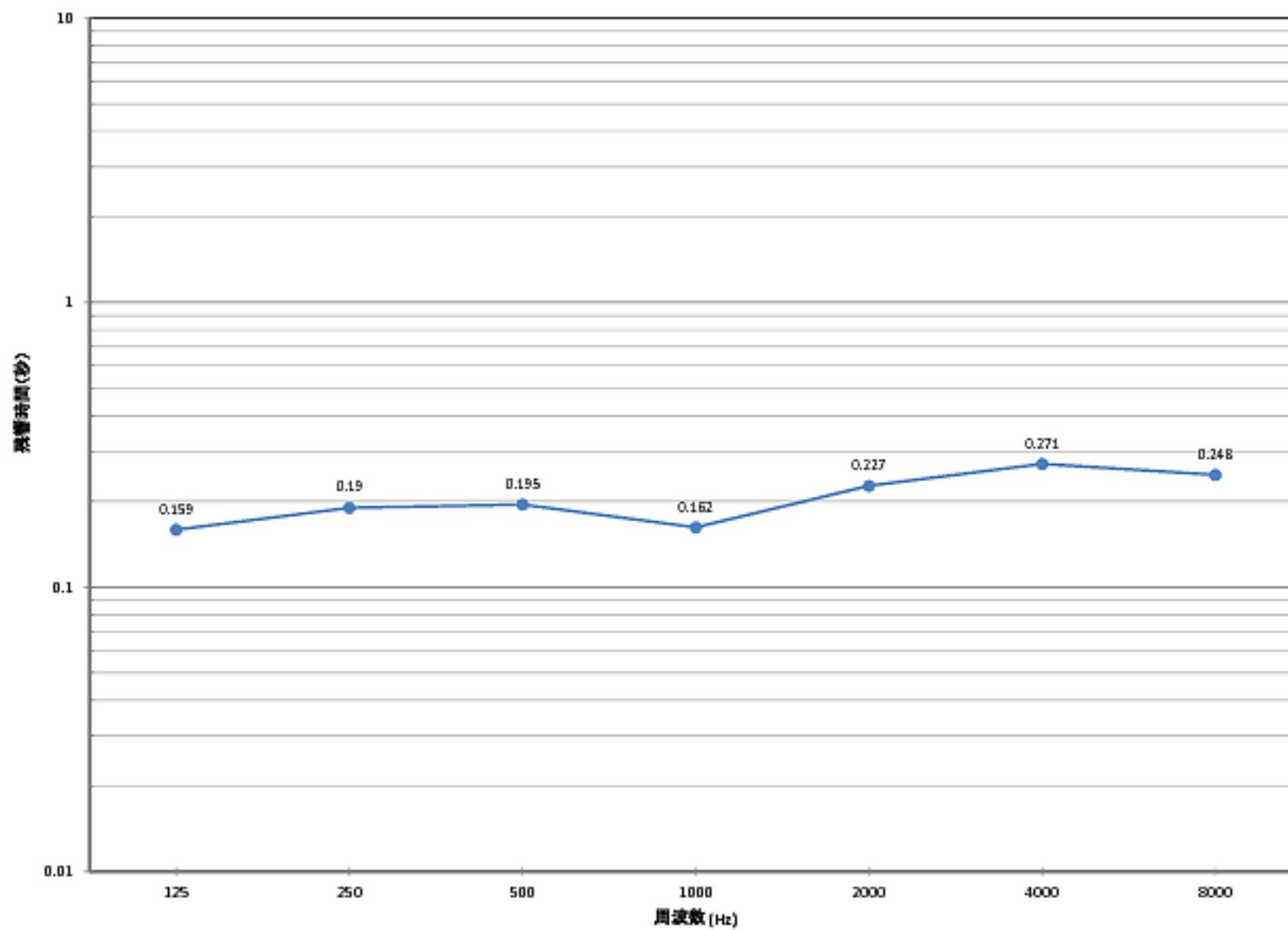
残響時間特性(測定位置 リスニングポイント)_HIRO Acoustic Model-CCCS
