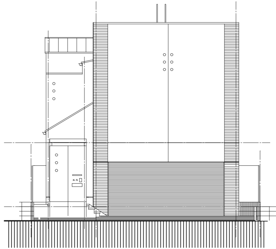
東立面图 1/100
