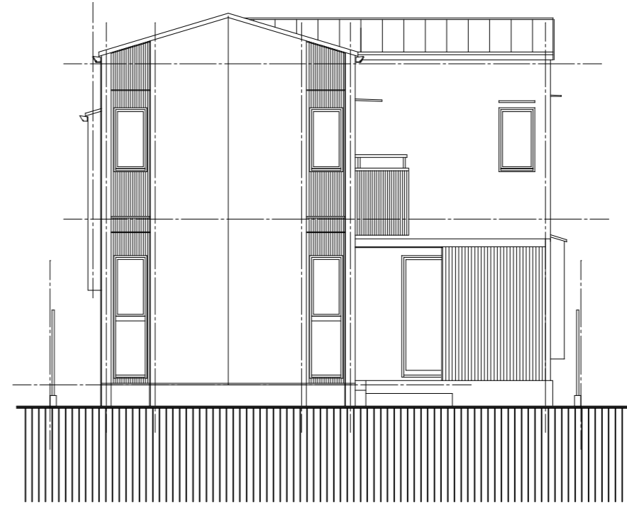
西立面图 1/100
