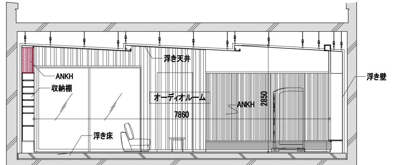
— 断面図(1) —
