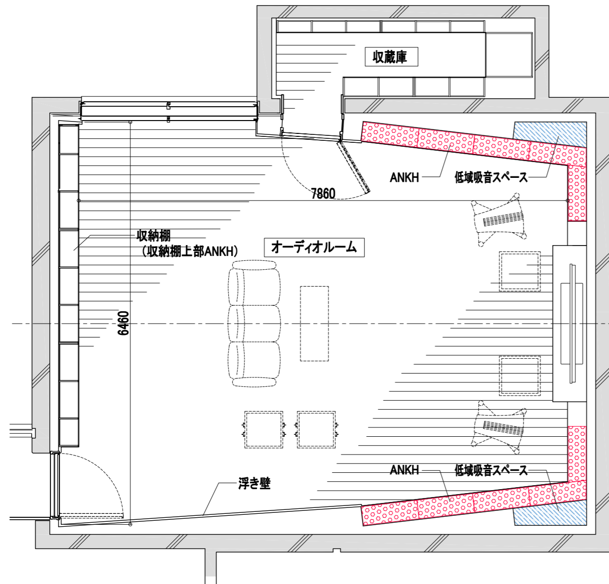
— 平面図 —
