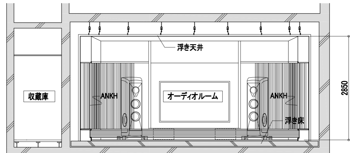
— 断面図(2) —
