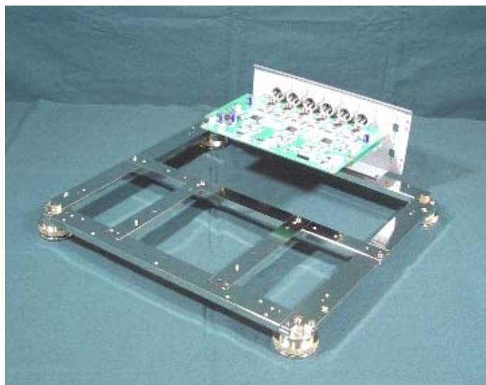
写真 12 リアパネルの取り付け
